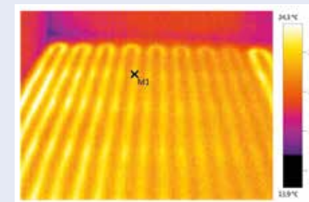
Fase di riscaldamento iniziale con risparmio energetico con il sistema RÖFIX SofoPlan® Slim (ripreso con telecamera a raggi infrarossi)
